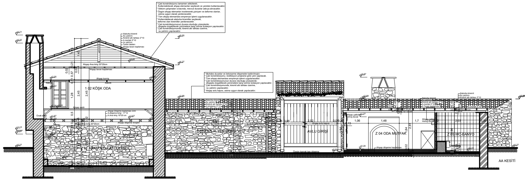
A-A KESİTİ
