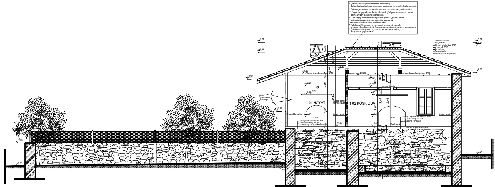
B-B KESİTİ
